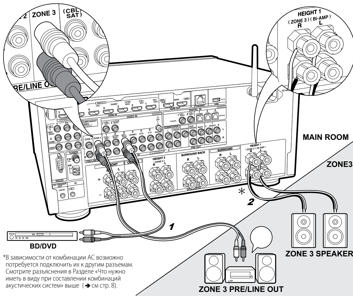
1 Аналоговый аудио кабель, 2 Колоночный кабель
