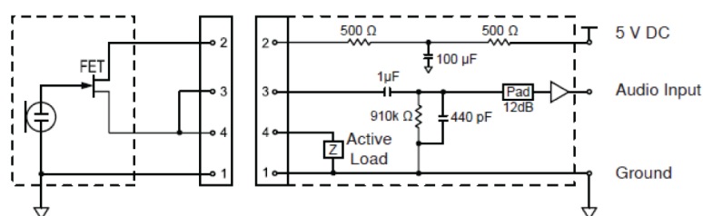
TA4M Connector
