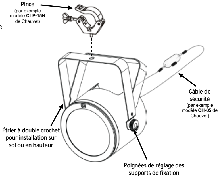
Schéma de montage
