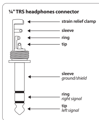
Рис. 8.2: Разъем наушников
