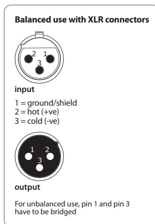
Рис. 8.1: XLR-соединения
