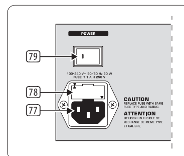
рис. 2.9: Секция POWER
