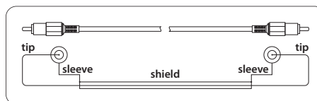
Рис. 8.3: RCA-кабель
