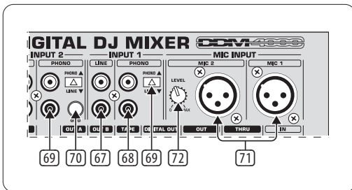
Рис. 2.7: Входы DDM4000
