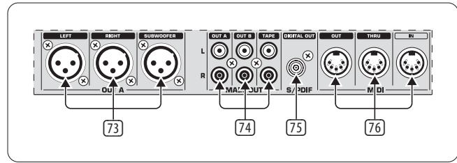
Рис. 2.8: Выходы DDM4000
