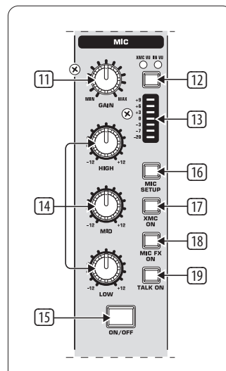
Рис. 2.2: Микрофонный канал
